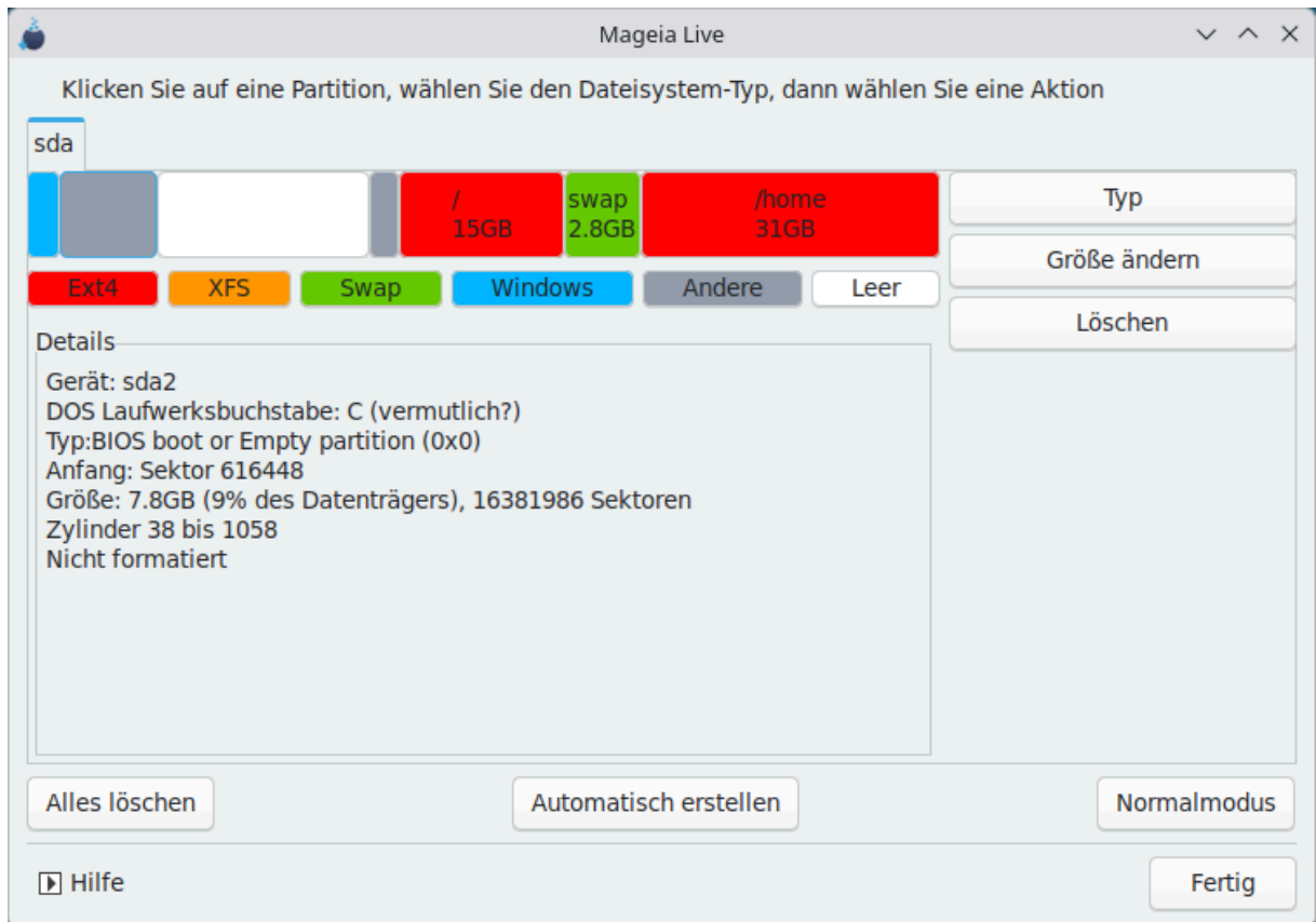
Abbildung 2. BIOS-Bootpartition
