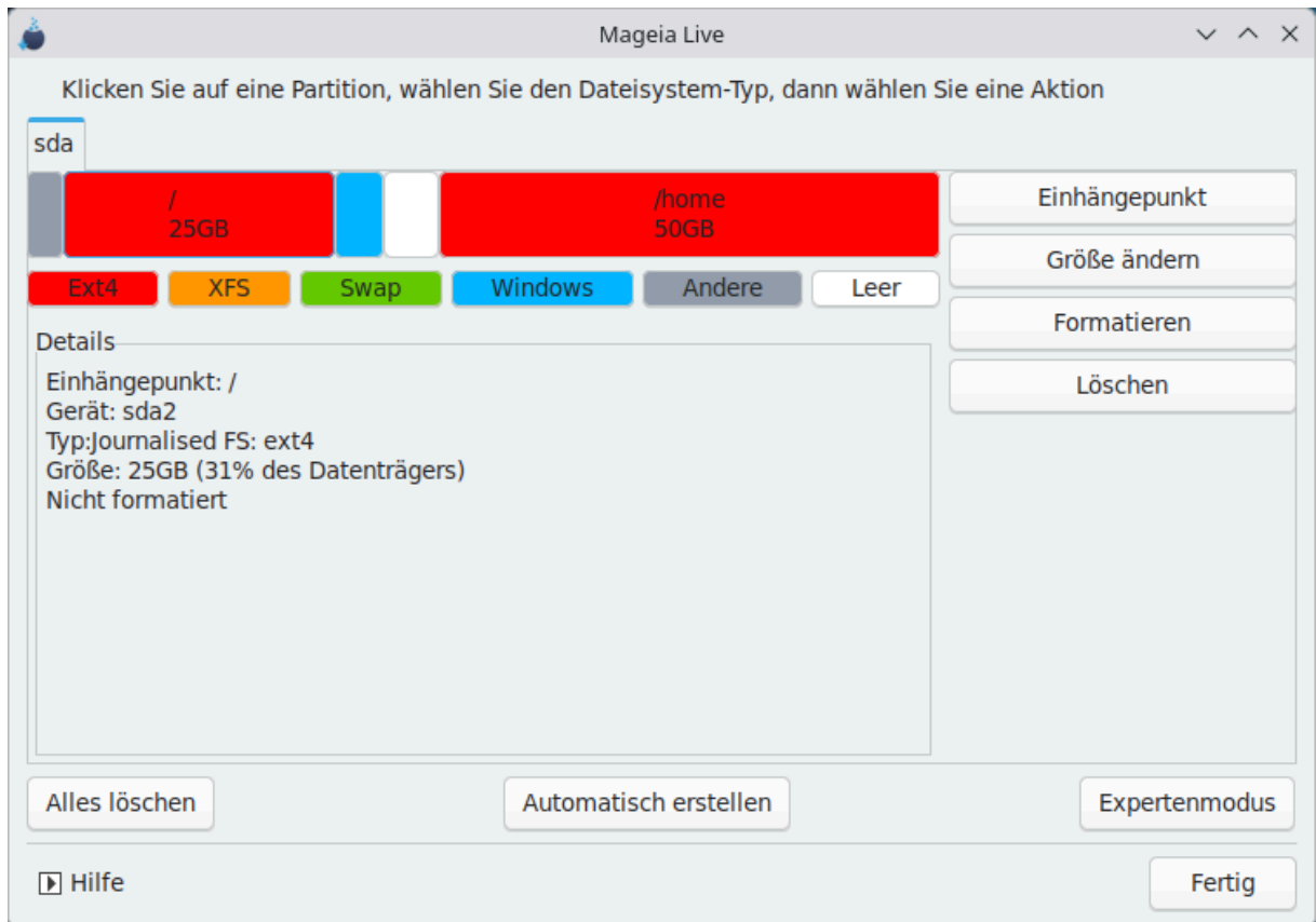
Abbildung 1. EFI-Systempartition
