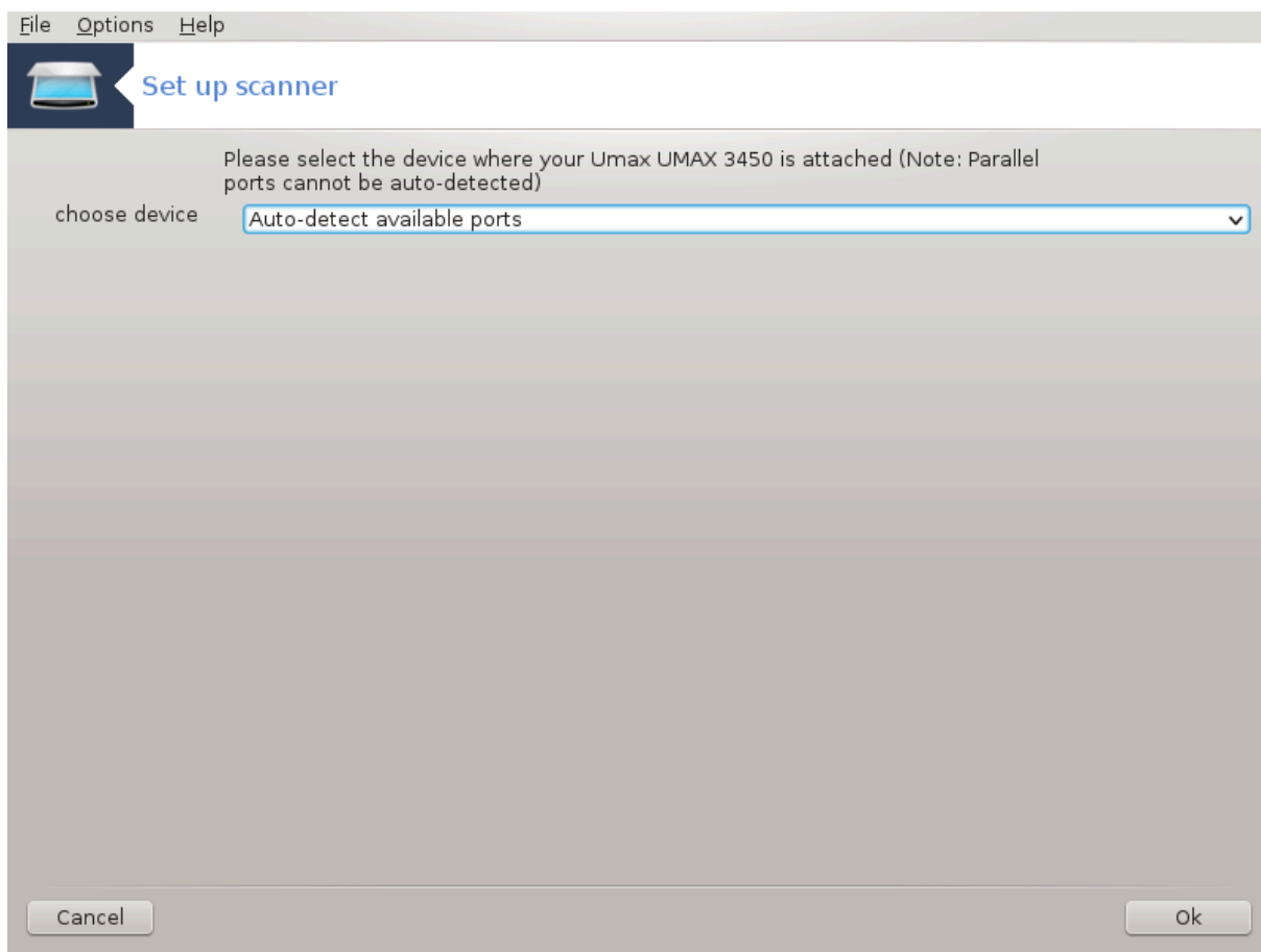
Slika 1. Choose port
